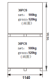
パレット合計：72枚 パレット正面図
