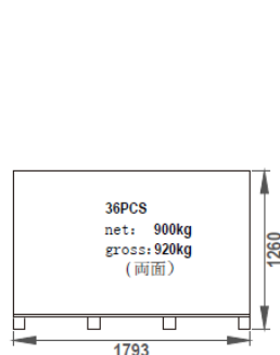
パレット単体：36枚 パレット側面図
