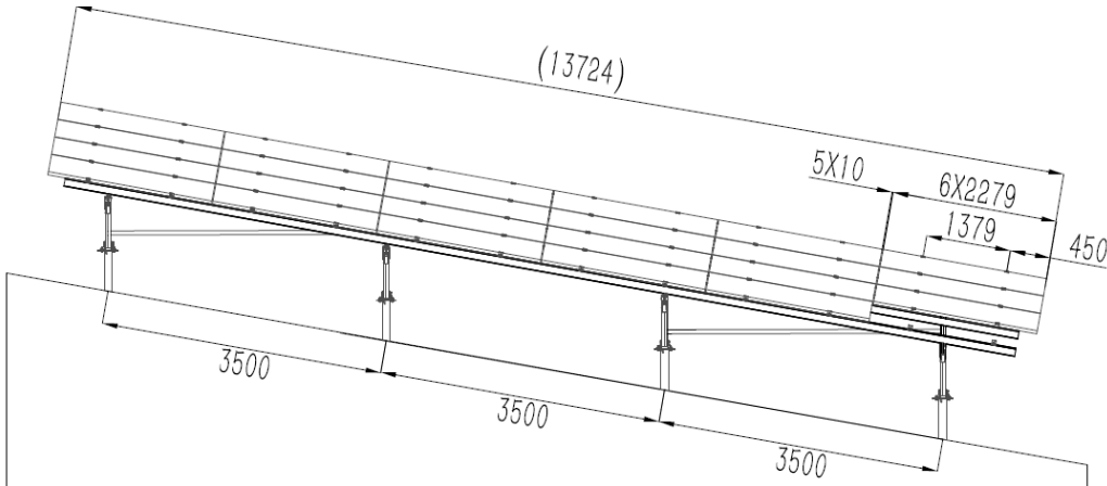
正面図
