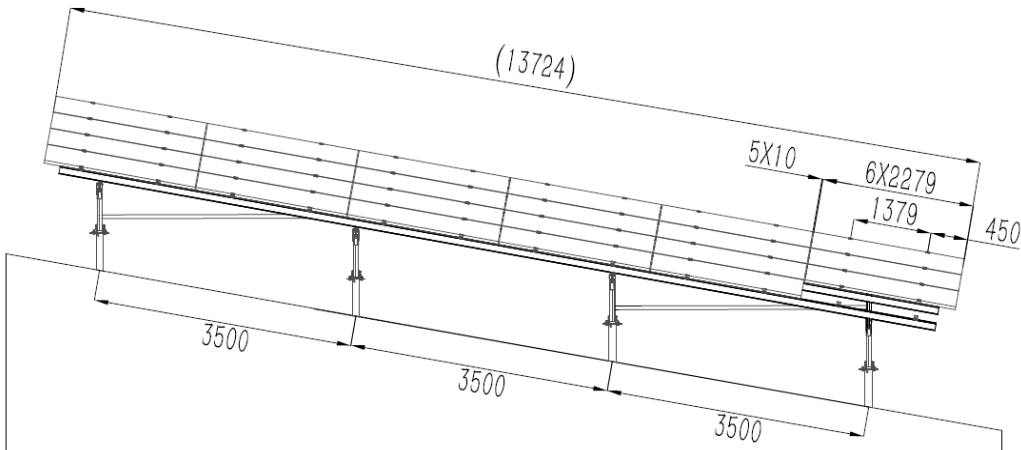
正面図
